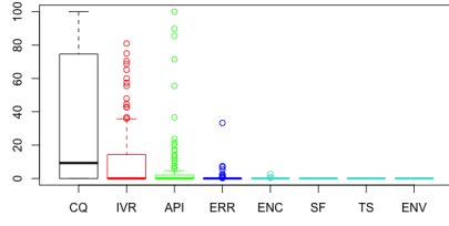
(d) Remained Warnings in the PVS-Studio
